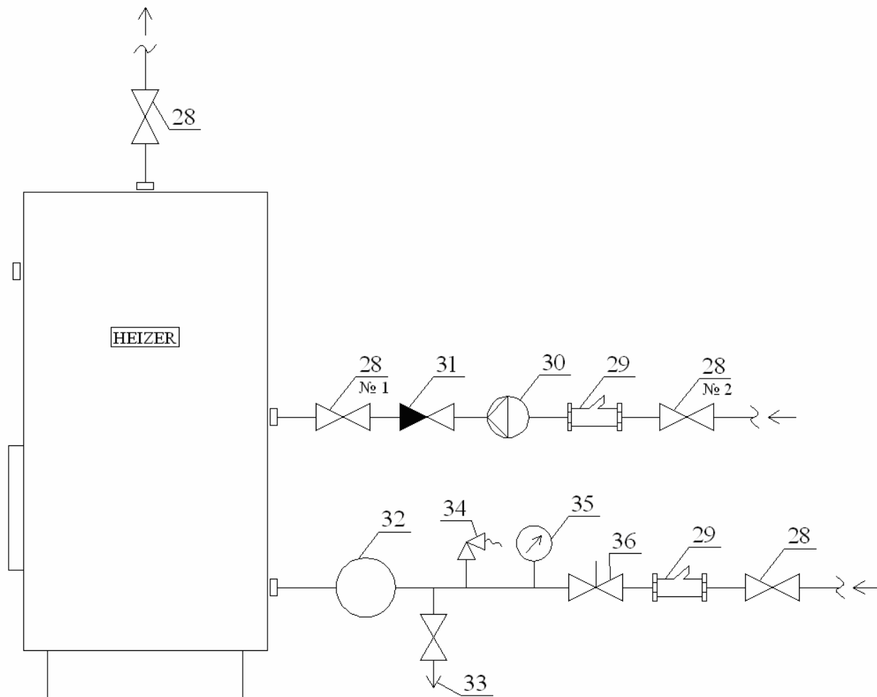
Рис. 1. Схема подключения электроводонагревателя Heizer Серии E
