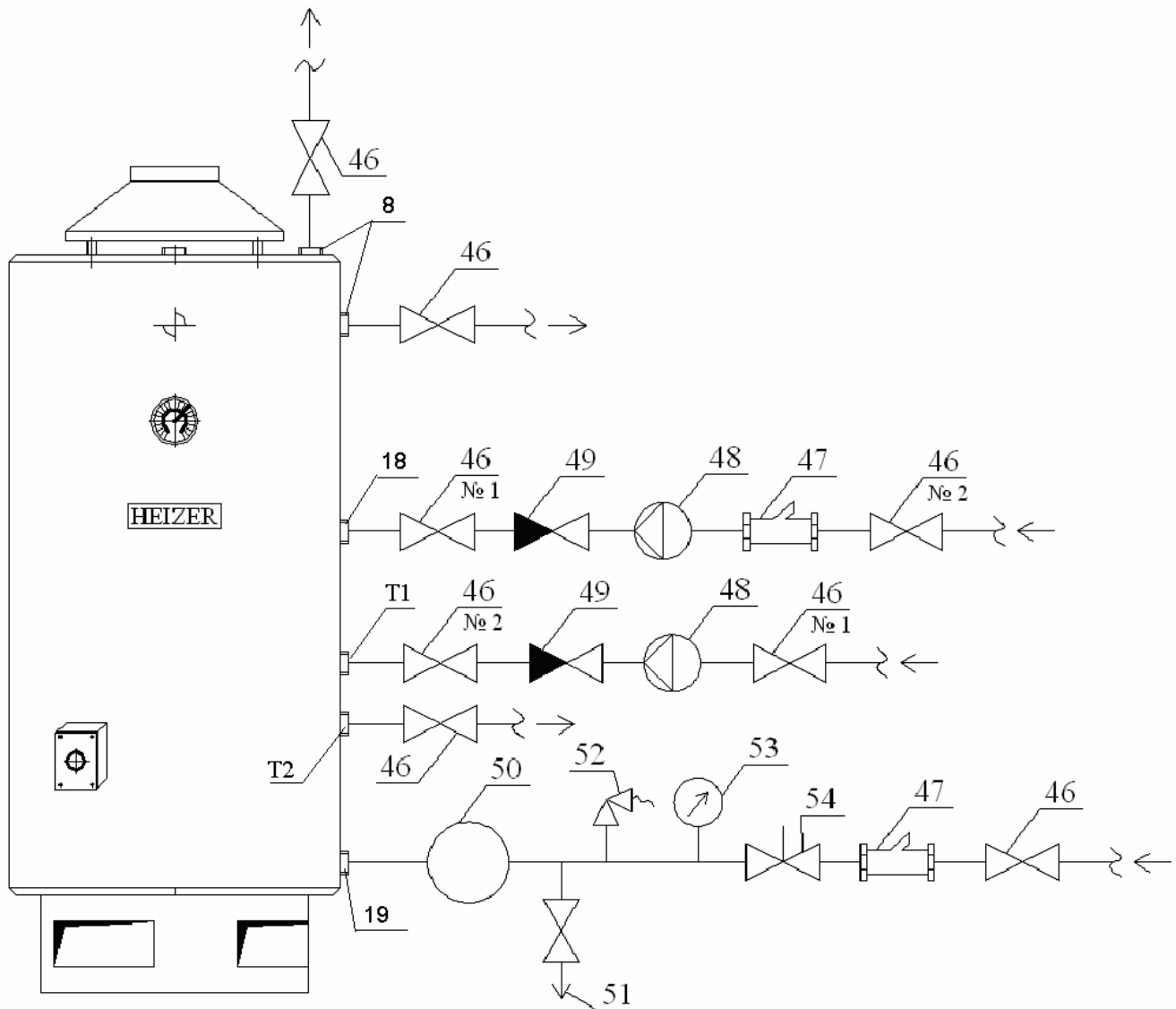
Рис. 1. Схема подключения газового водонагревателя Heizer Серии GT
