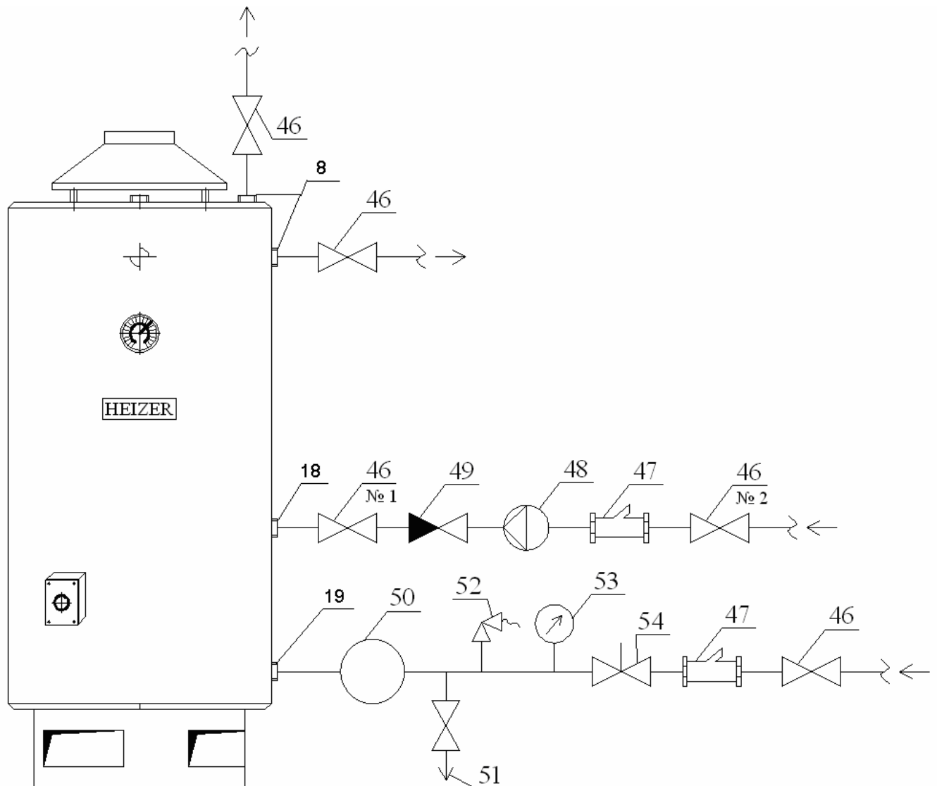
Рис. 1 Схема подключения напольного газового водонагревателя
