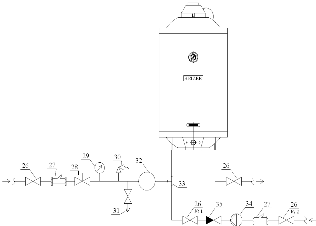
Рис. 1. Схема подключения навесного газового водонагревателя Heizer Серии GAN
