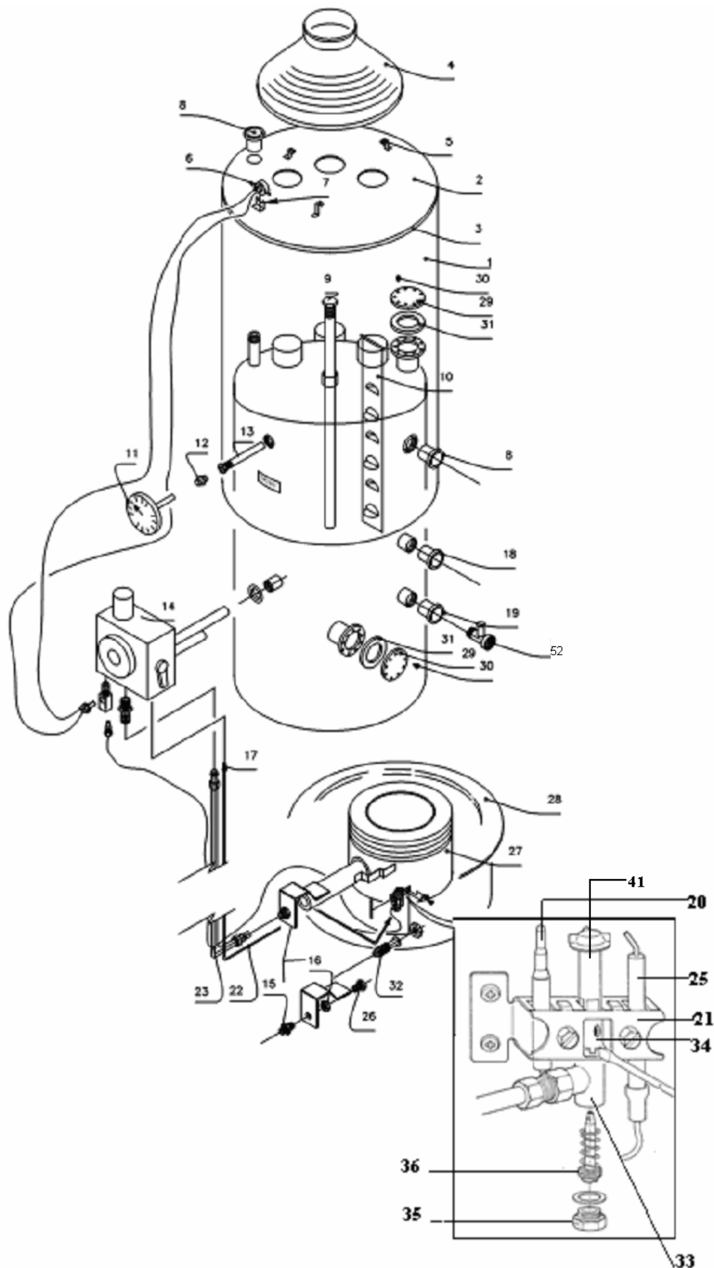
Рис. 1 Подробная схема водонагревателя
